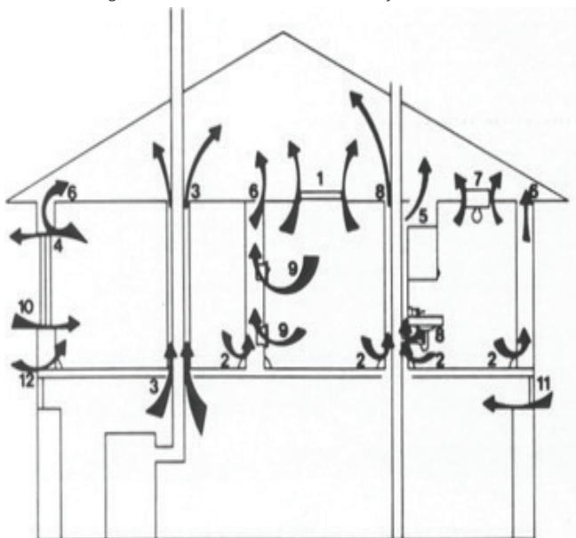
Slika 1: Pogosta mesta nekontrolirane izmenjave zraka
